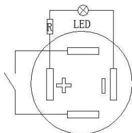
电气简图
