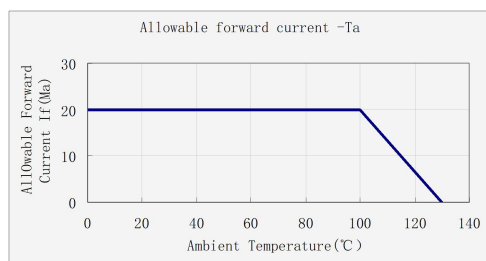
最大正向直流电与温度曲线图 Maximum Forward DC vs. Temperature Graph
