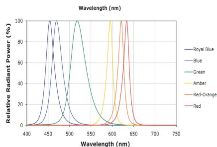
波长特征 Wavelength characteristics
