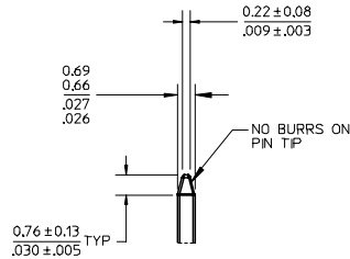
DETAIL Y SCALE 5:1
