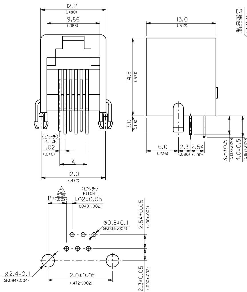
基板穴推奨寸法 RECOMMENDED P.C.B. LAYOUT (ジャック取付け側) (JACK ASS'Y SIDE)
