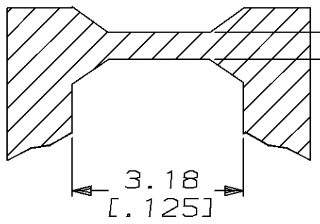
SECTION A-A SCALE 10:1
