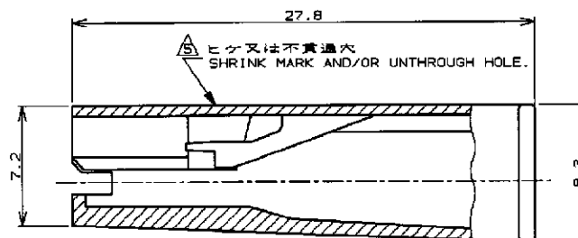
断面 "A" - "A" (SECT "A" - "A")
