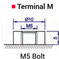
M5 Bolt & Nut
