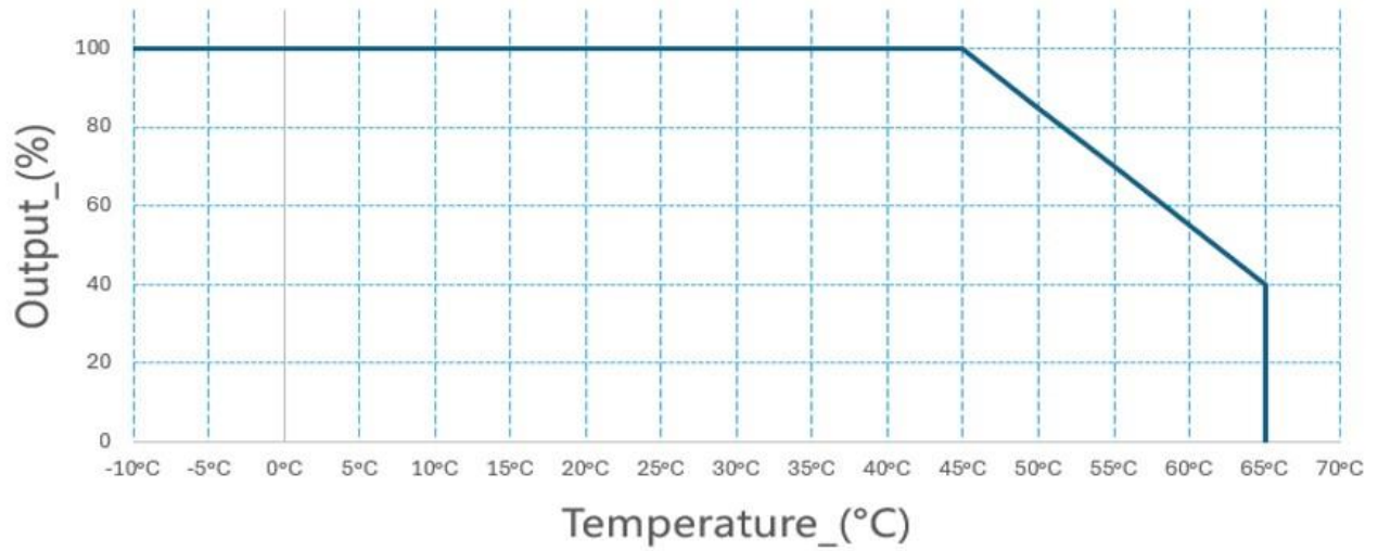
【36W_Derating Curve】
