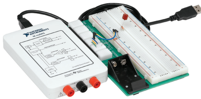
▲ NI myDAQ
