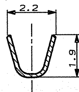
SEZ. (SECT.) D-D
