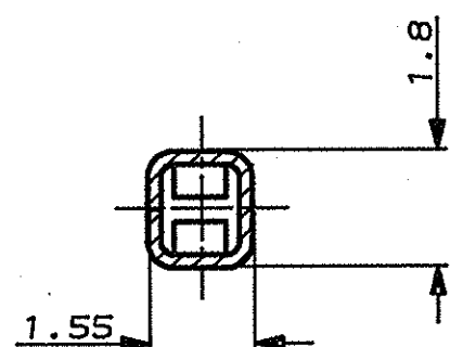
SEZ. (SECT.) A-A
