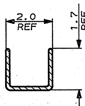
SEZ. (SECT.) E-E
