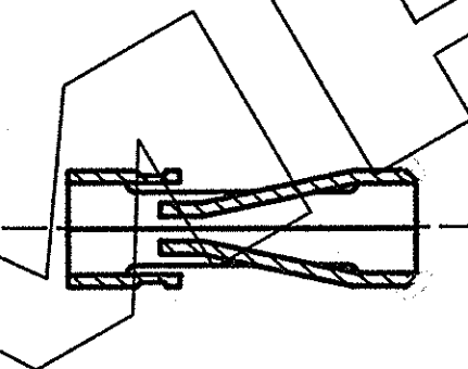
SEZ. (SECT.) B-B
