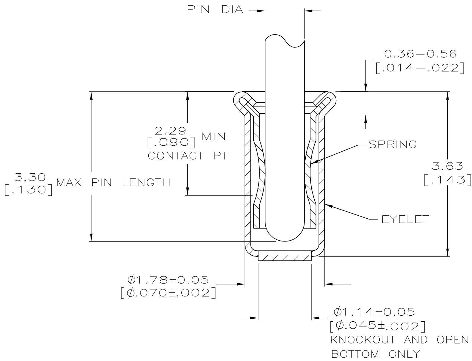
SECTION A-A
