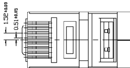
#T8TR : MP8P8C R.SHD
