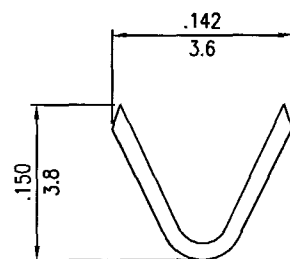
A-A SECTION
