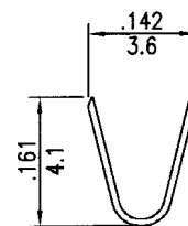
A-A SECTION
