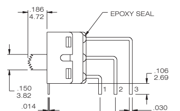
TS-13L-A1-2-Q(-E)
