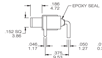
TS-13P-A1-2-Q(-E)
