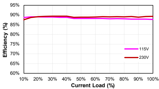
TRH70A360 (Eff Vs Io)
