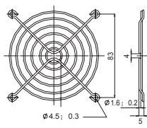
FG-09 For 92mm Fan
