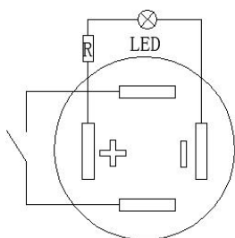
电气简图
