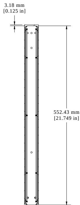
SECTION A-A
