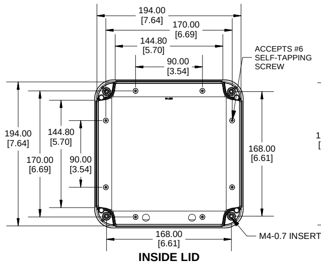
INSIDE LID
